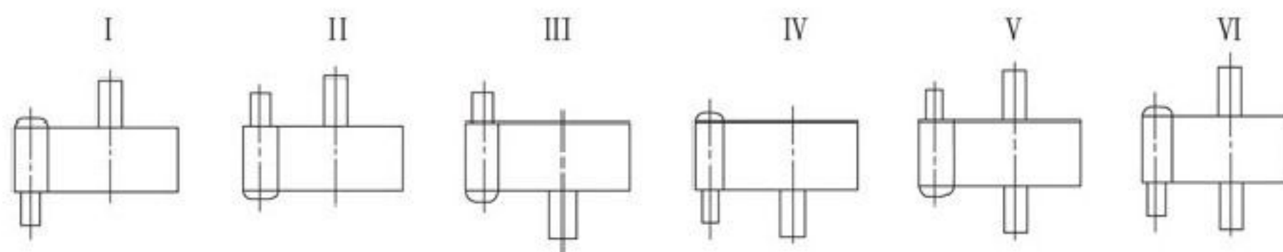
装配型式
