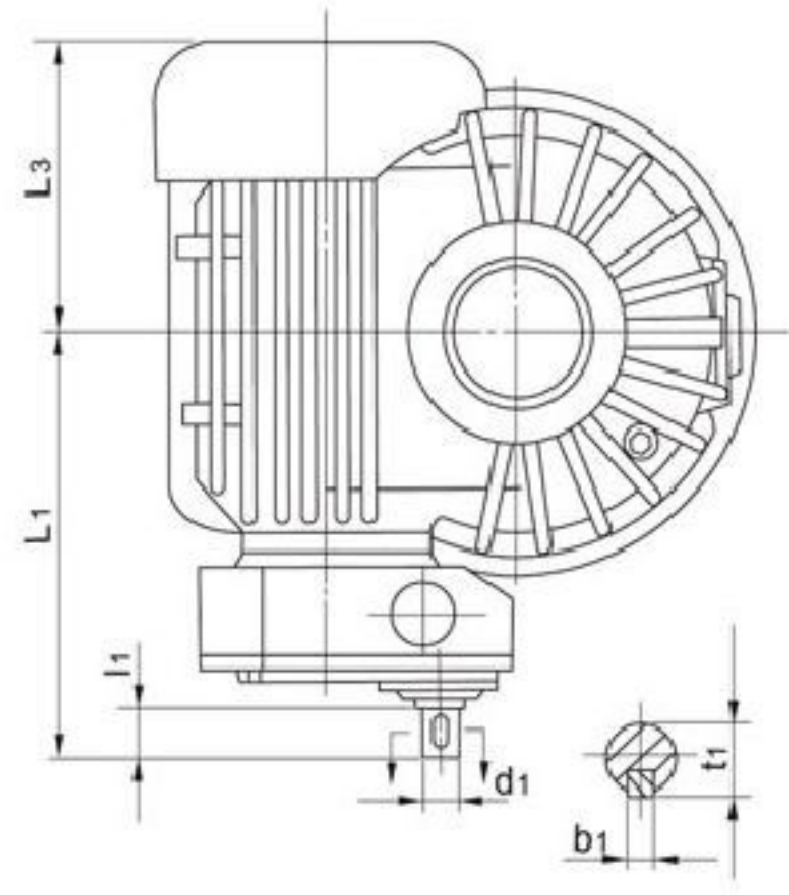
装配型式
